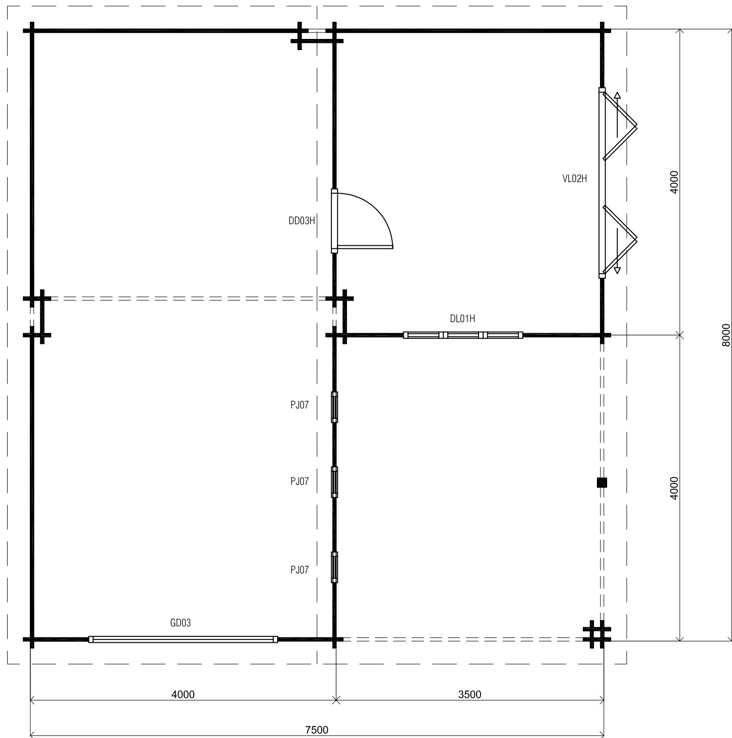
Plattegrond / Plan
